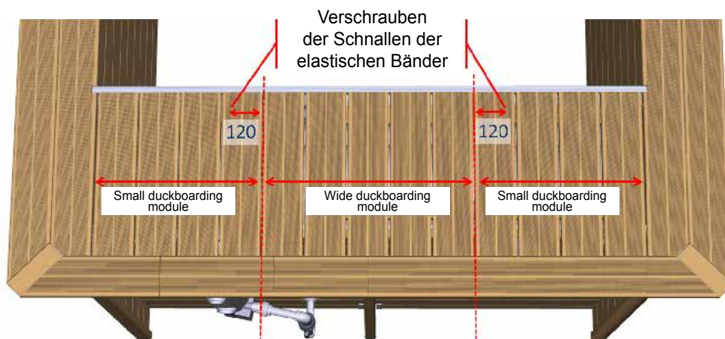
Abbildung 52 – Anbringen der elastischen Bänder unter den Holzrosten
