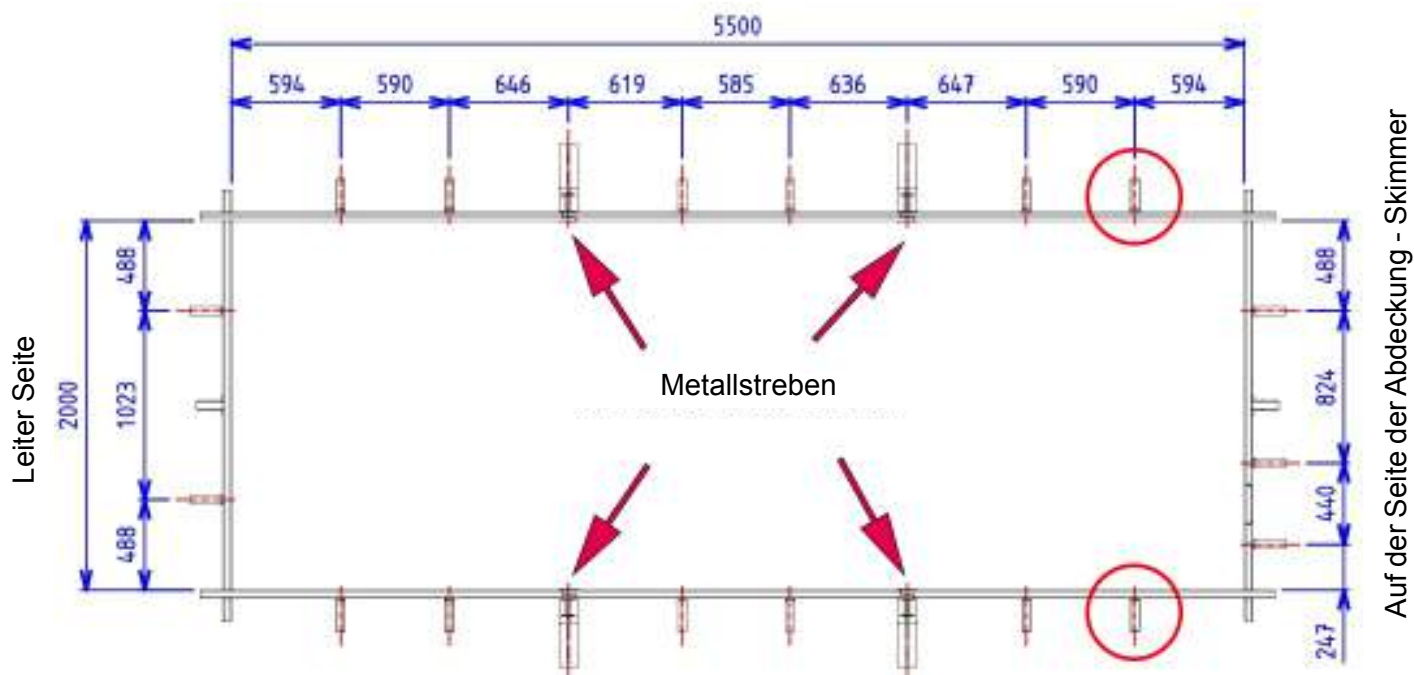
Abbildung 15 – Lage der Holzkeile des Handlaufs
