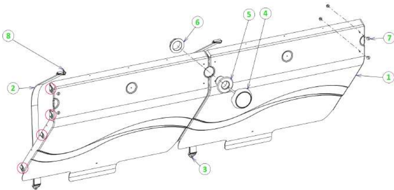
Abbildung 42 – Montage der Trennwand und des Projektors
