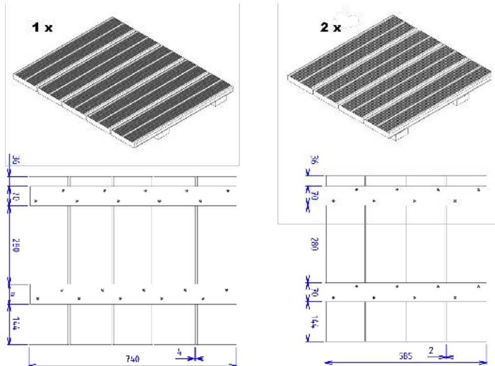
Abbildung 51 – Montage der Holzroste
