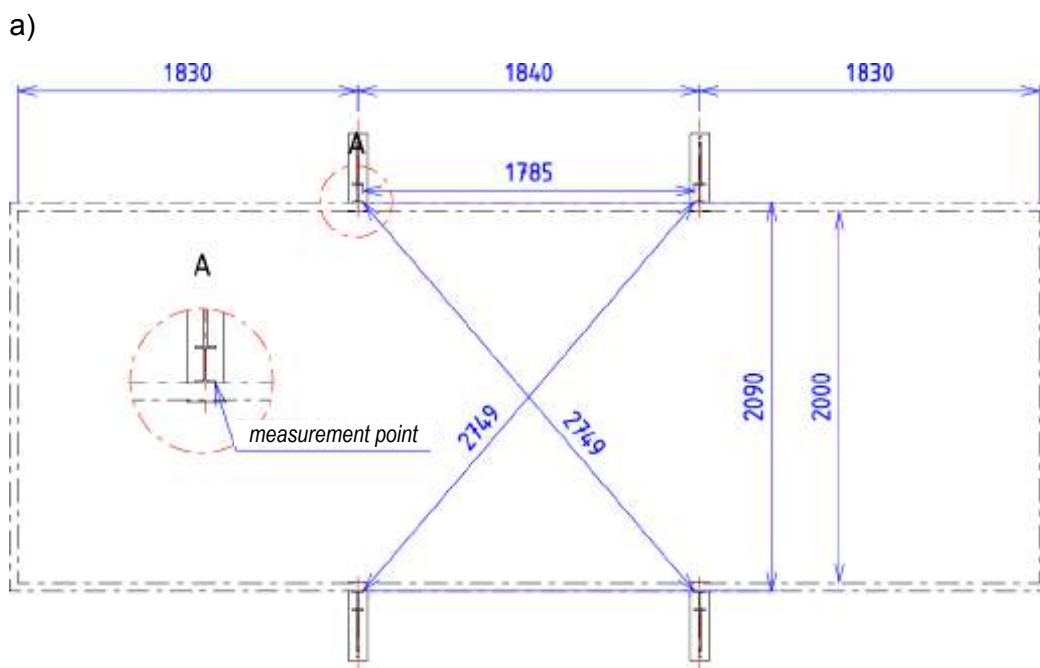
b) Abbildung 4 – a und b - Positionierung der Strebe
